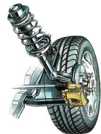
Sicherheitsfahrwerk mit Gasdruck-Stoß- dämpfern und -Feder- beinen.
