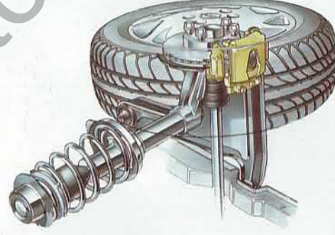
Sicherheitsfahrwerk mit Gasdruck-Stoß- dämpfern und -Feder- beinen.
