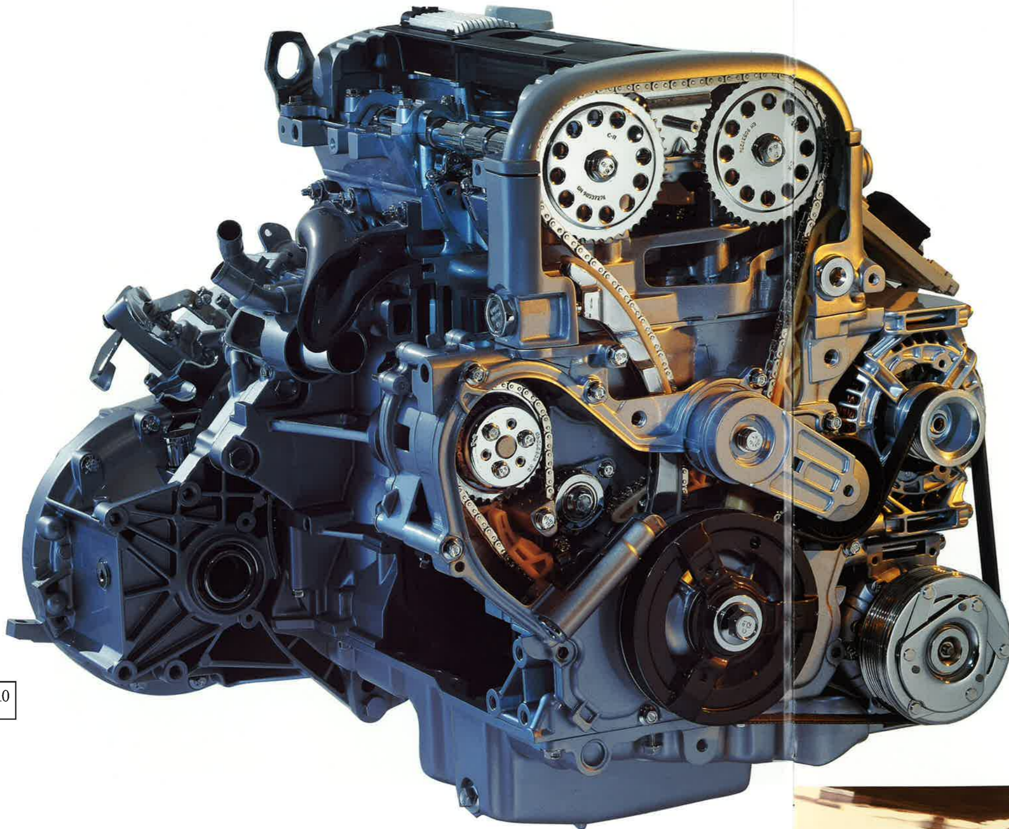
■ Sportliches Leichtgewicht. Der neue 2.2 16V ECOTEC-Motor (lieferbar voraussichtlich ab Mai 2000).
