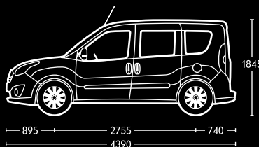
Combo mit Radstand L1 und Dachhöhe H1.
