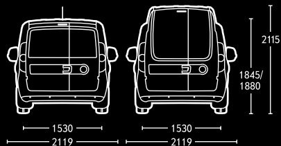
Combo mit Dachhöhe H1 oder H2.
