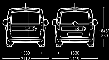
Kastenwagen mit Heckflügeltüren oder Heckklappe.
