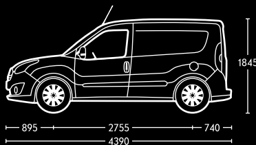
Kastenwagen mit Radstand L1 und Dachhöhe H1.
