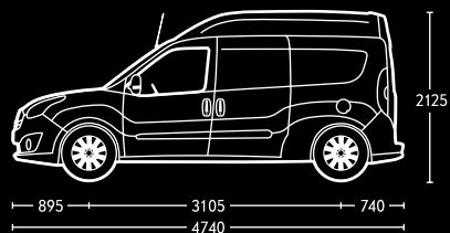
Kastenwagen mit Radstand L2 und Dachhöhe H2.
