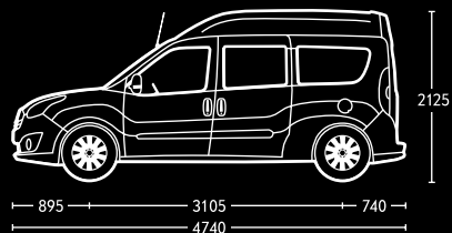
Kastenwagen verglast mit Radstand L2 und Dachhöhe H2.
