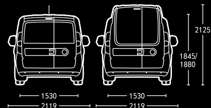
Kastenwagen mit Dachhöhe H1 oder H2.
