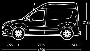
Kastenwagen mit Radstand L1 und Dachhöhe H2.
