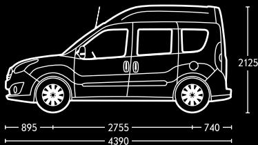
Kastenwagen verglast mit Radstand L1 und Dachhöhe H2.
