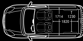
Kastenwagen mit Radstand L1 und Dachhöhe H1 oder H2.
