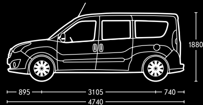
Kastenwagen verglast mit Radstand L2 und Dachhöhe H1.
