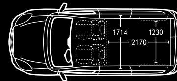
Kastenwagen mit Radstand L2 und Dachhöhe H1 oder H2.
