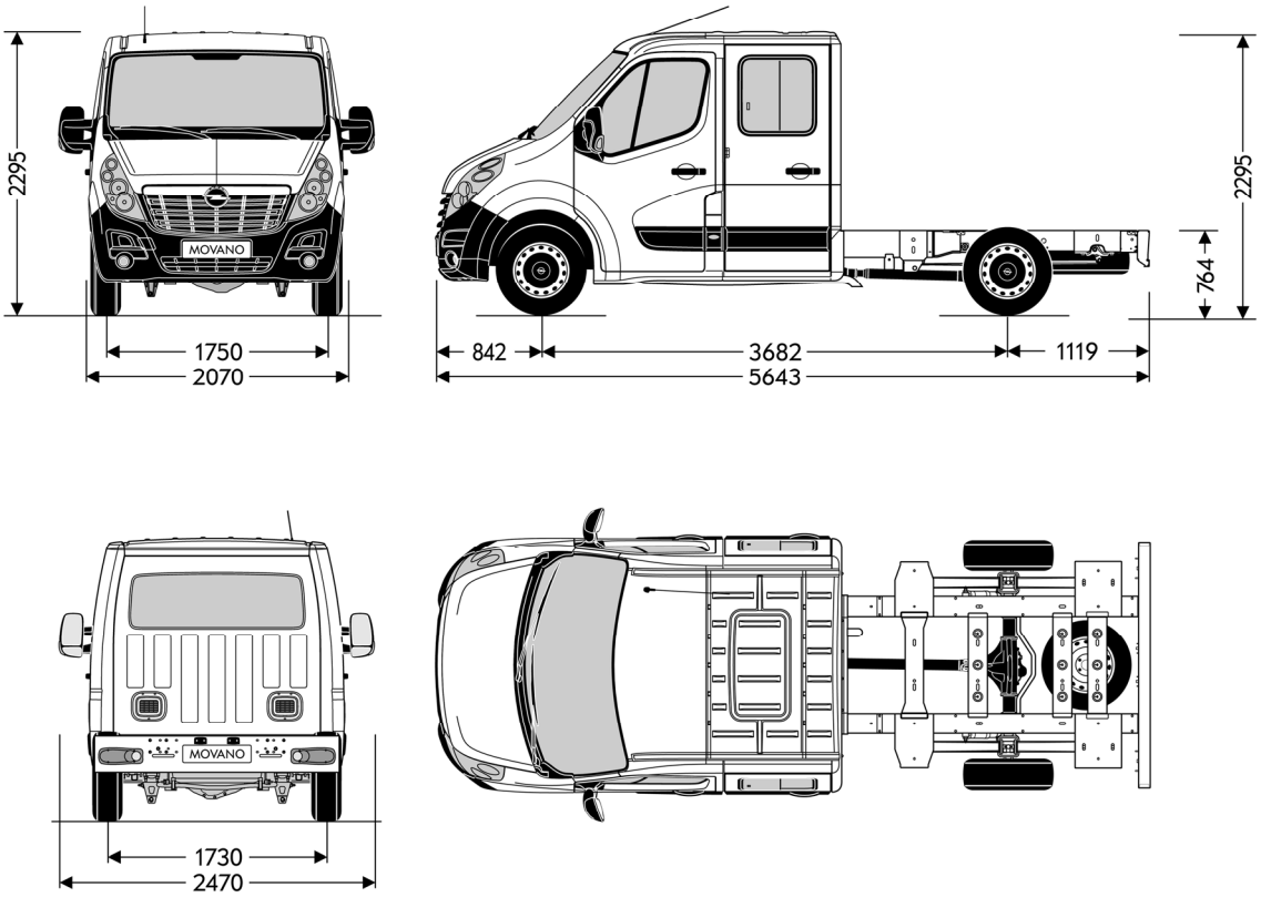
L2H1 Alle Maße in mm
