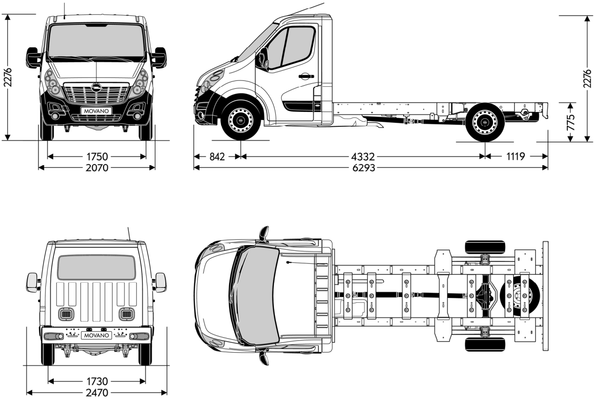
L3H1 Alle Maße in mm
