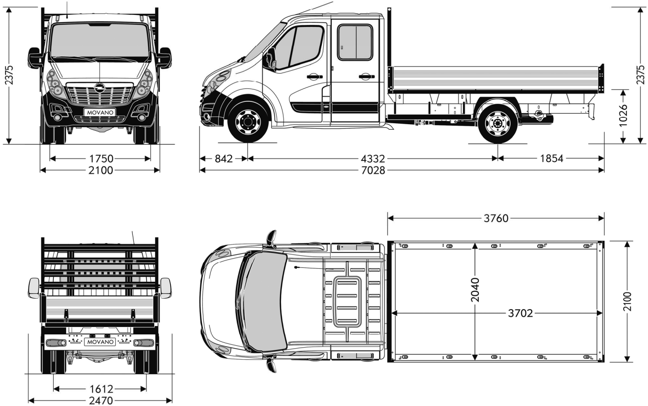
L4H1 Alle Maße in mm
