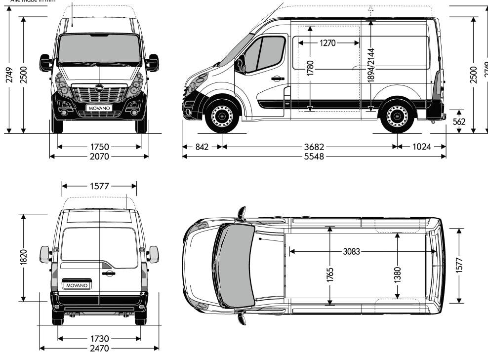
L2H2-3 Alle Maße in mm
