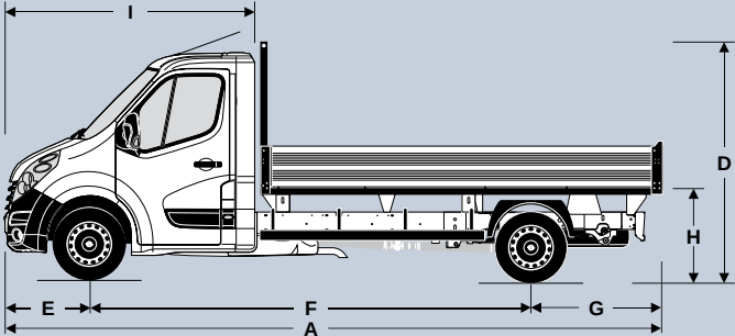
Pritsche Einzelkabine: Abmessungen
