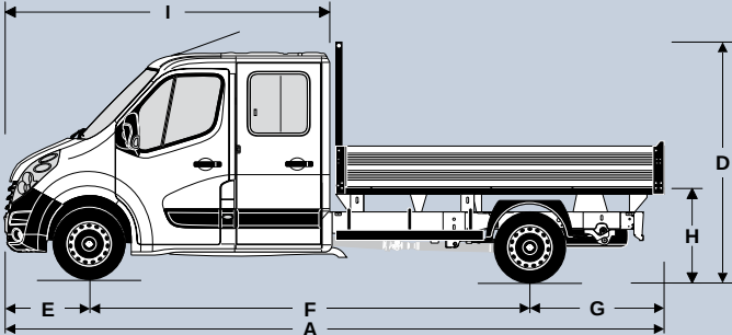
Pritsche Doppelkabine: Abmessungen
