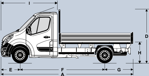
Kipper Einzelkabine: Abmessungen
