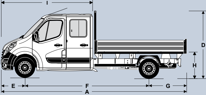
Kipper Doppelkabine: Abmessungen
