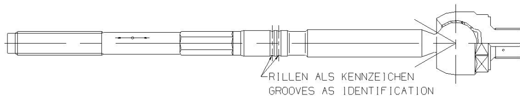
Spurstange mit den zwei Rillen als Kennzeichnung
