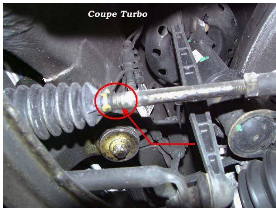
Spurstange im eingebauten Zustand
