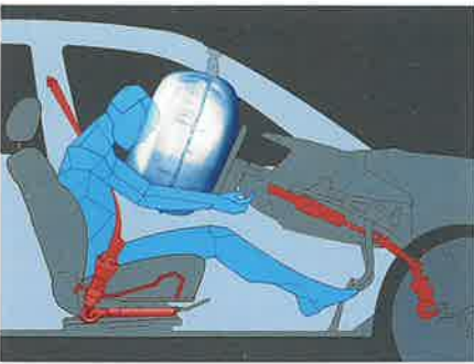
Die pyrotechnischen Gurtstraffer und Airbags werden synchron von der Single Sensing Unit aktiviert.
