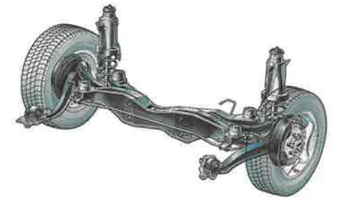
Die Multi-Link-Hinterachse erhöht die Spurstabilität und die Lenkpräzision. Durch die Lagerung auf einem isolierten Quertträger werden zudem Fahrgeräusche und Vibrationen entscheidend vermindert.
