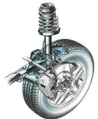
Die Vorderräder des Vectra werden über Gasdruckfederbeine mit Querlenker und Stabilisator geführt und sind individuell auf das jeweilige Modell abgestimmt.
