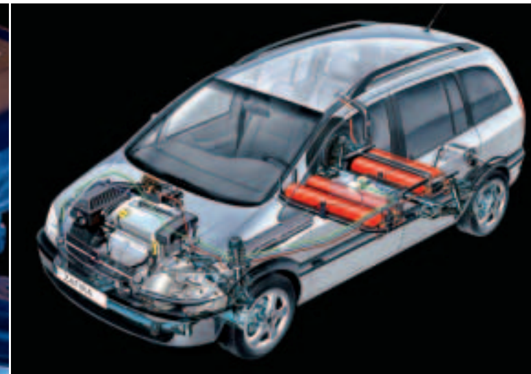
Besonders umweltschonend: der Zafira 1.6 CNG mit Erdgasantrieb. Mit 71 kW (97 PS) und einem maximalen Drehmoment von 140 Nm ist er sparsamer, aber fast genauso leistungstark wie sein benzinbetriebenes Pendant.
