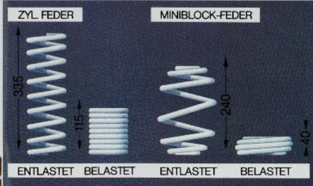
Miniblockfedern
