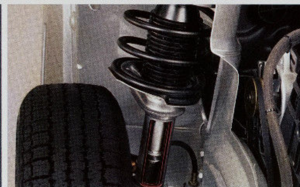
Federbein-Vorderrad-Aufhängung nach dem McPherson-Prinzip
