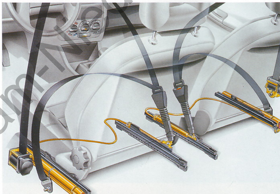
Blitzschnell zieht der Gurtschloßstraffer – und nicht mehr der Gurtaufrollautomat – des Aktivgurt-Systems bei einem Frontalaufprall die Gurte an. Die Vorwärtsbewegung von Fahrer und Beifahrer wird weitgehend reduziert.
