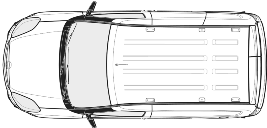
Breite mit eingeklappten Außenspiegeln 1850 mm
