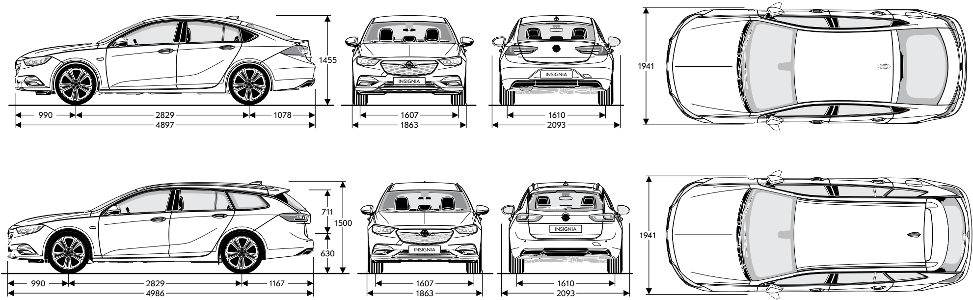
Breite mit eingeklappten Außenspiegeln 1941 mm
