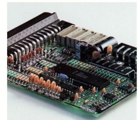
Die Elektronik der Fahrwerksdämpfung denkt mit. Ab 115 km/h schaltet sie bei „Komfort“-Einstellung automatisch auf „normal“.
