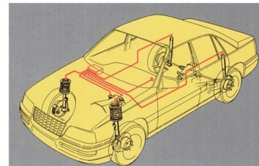
Kleine Stellmotoren in den Stoßdämpfern drehen entsprechend der Geschwindigkeit oder der manuellen Einstellung einen Kolben mit unterschiedlich großen Öffnungen.
