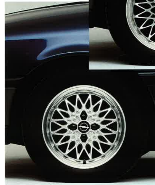
Leichtmetallrad, 1750317, 6J x 15, mit ABE, felgenhornkopiert. Farbe: Silber, Zierkappe für Radnabe und Abdeckkappen für Radschrauben.
