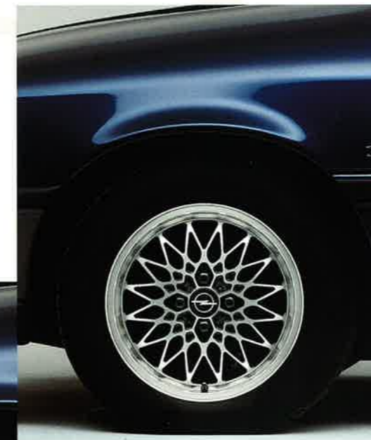
Leichtmetallrad, 1750317, 6J x 15, mit ABE, felgenhornkopiert. Farbe: Silber, Zierkappe für Radnabe und Abdeckkappen für Radschrauben.
