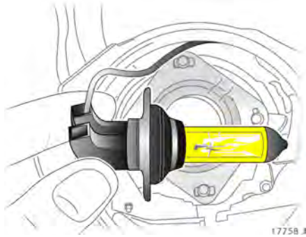
5. Lampenträger mit Glühlampe aus Reflektor nehmen.
