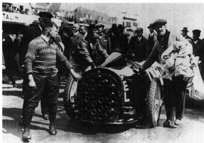
Heißes Hinterteil: Der Rak 2 war ein wahrlich explosives Gefährt
