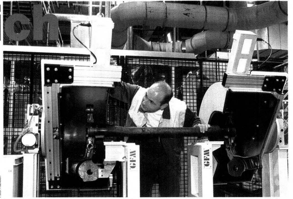
Drum prüfe, wer sich ewig bindet: Rolf Schlotzhauer checkt den Versatz am Torsionsprofilrohr
